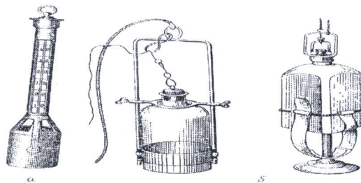
Мал. 16.1. Термометр для вимірювання температури води в водоймах, колодязях (а), батометри для відбору проб води на аналіз (б).
