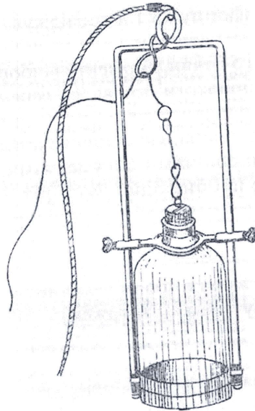
Рис. 2 . Батометр
