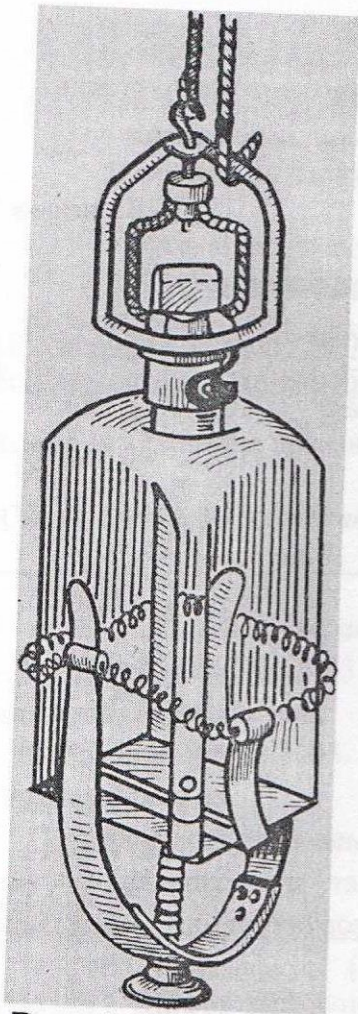
Рис. 1 . Батометр
