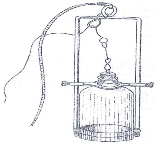
Рис. 2 . Батометр
