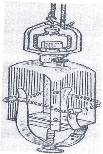
Рис. 1 . Батометр
