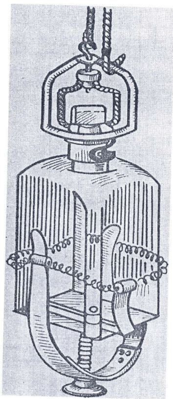
Рис. 1 . Батометр
