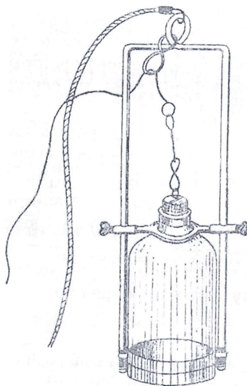
Рис. 2 . Батометр
