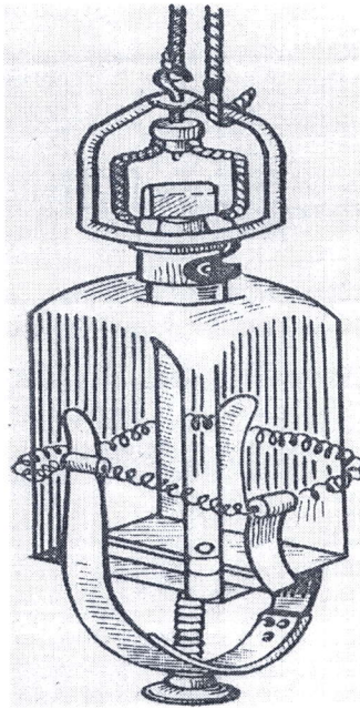
Рис. 1 . Батометр
