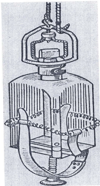
Рис. 1 . Батометр
