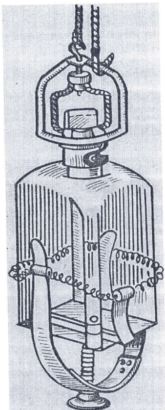
Рис. 1 . Батометр
