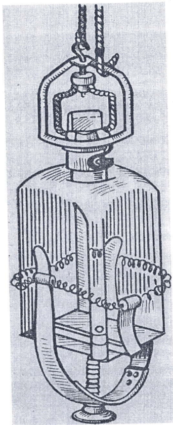
Рис. 1 . Батометр
