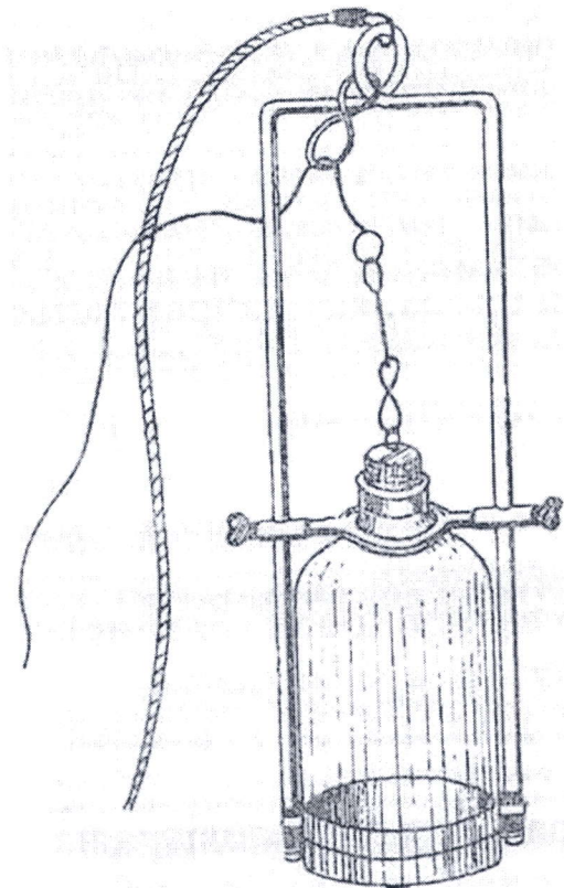
Рис. 2 . Батометр
