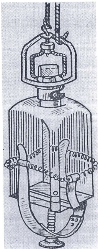
Рис. 1 . Батометр
