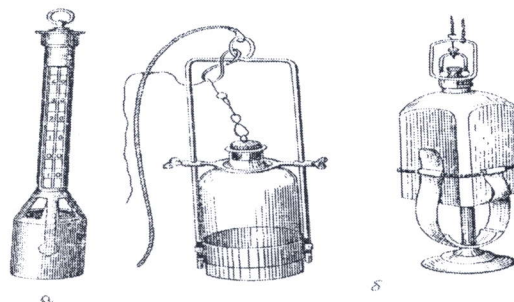
Мал. 16.1. Термометр для вимірювання температури води в водоймах, колодязях (а), батометри для відбору проб води на аналіз (б).
