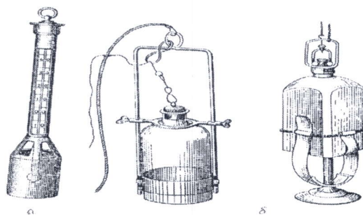
Мал. 16.1. Термометр для вимірювання температури води в водоймах, колодязях (а), батометри для відбору проб води на аналіз (б).
