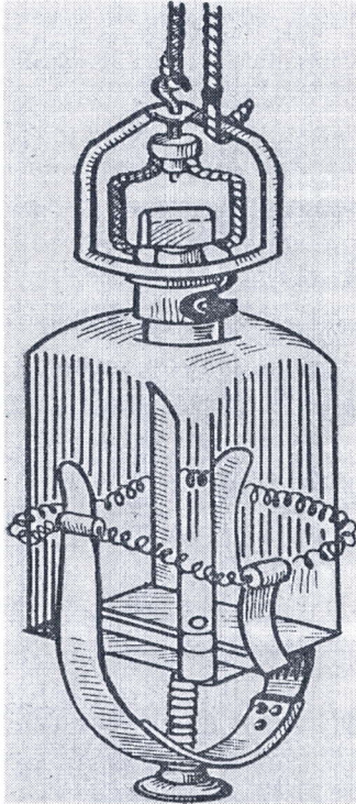
Рис. 1 . Батометр
