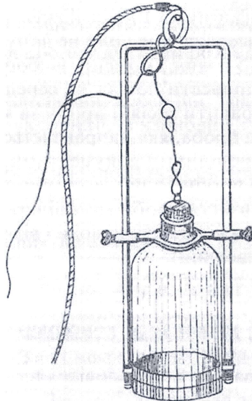
Рис. 2 . Батометр
