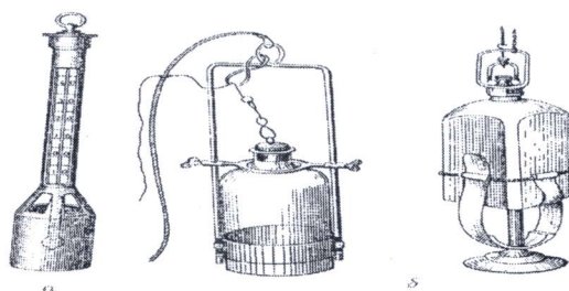
Мал. 16.1. Термометр для вимірювання температури води в водоймах, колодязях (а), батометри для відбору проб води на аналіз (б).
